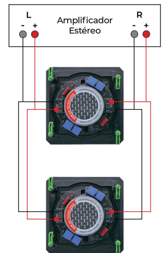
LIGAÇÃO DE 2 FALANTES POR ZONA
